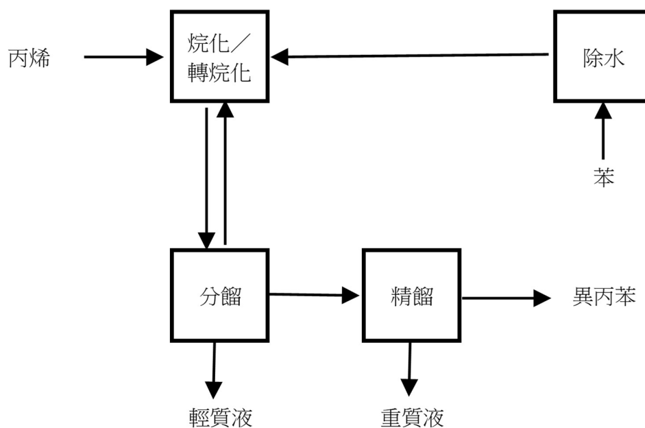
異丙苯生產流程（觸媒：沸石Zeolite）簡圖
