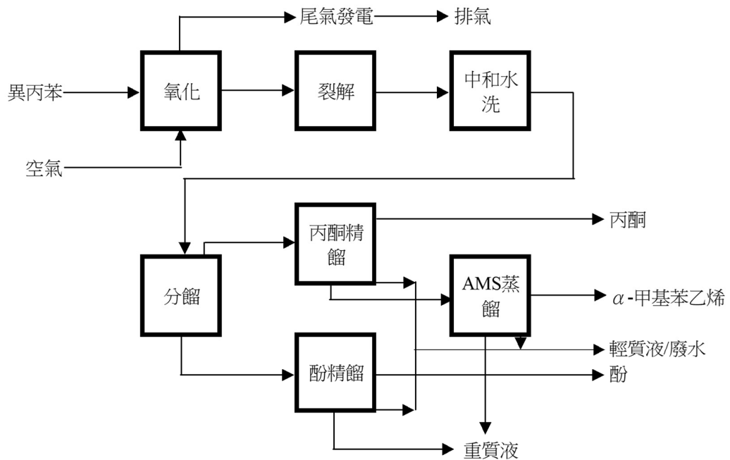
酚丙酮工場生產流程簡圖
