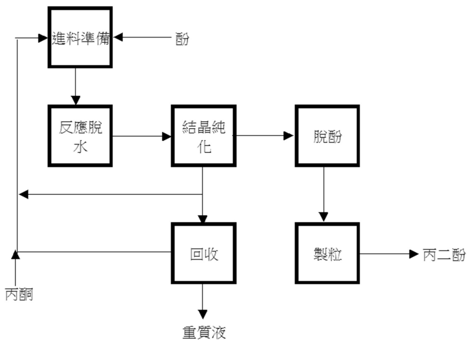
丙二酚生產流程簡圖
