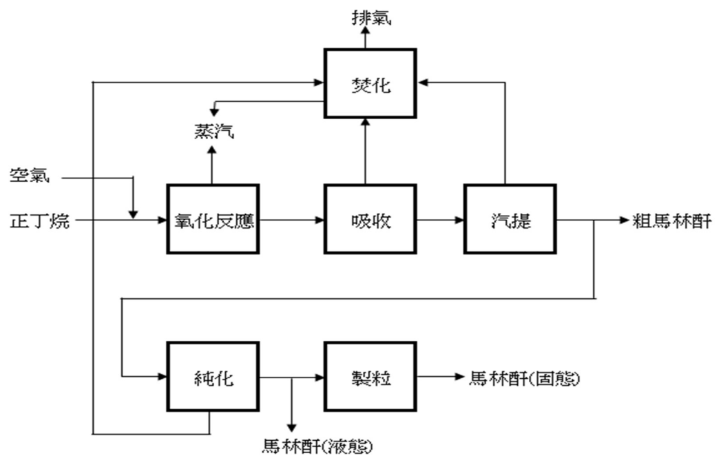
馬林酐工場生產流程簡圖
