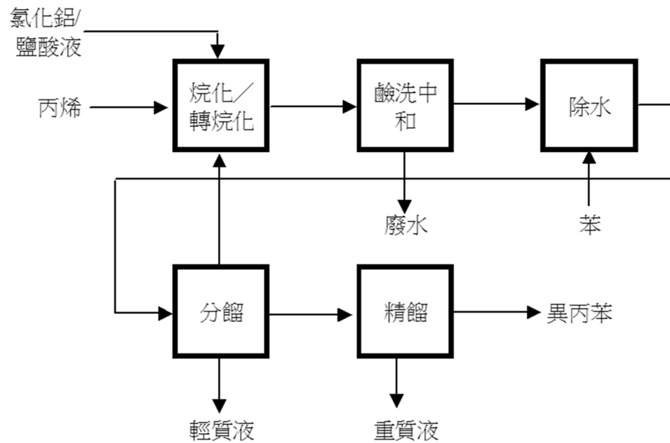
異丙苯生產流程(觸媒：氯化鋁鹽酸液)簡圖
